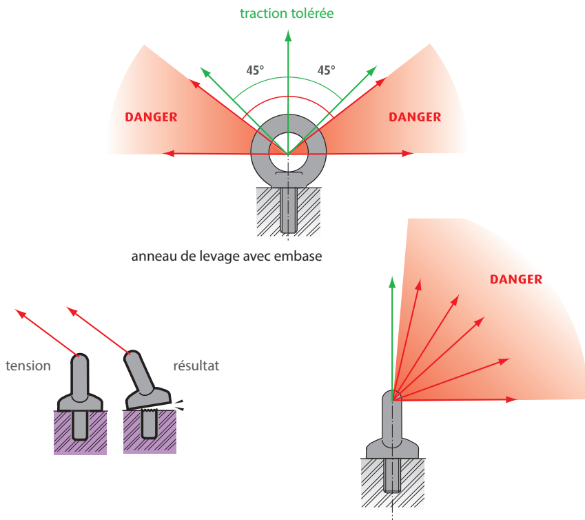
Figure 38 - Utilisation correcte des anneaux de levage
