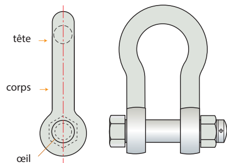
Figure 18 a - Manille lyre avec axe de type à vis à tête hexagonale, écrou hexagonal et goupille fendue
