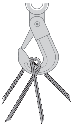
Figure 41 e - Brins superposés
