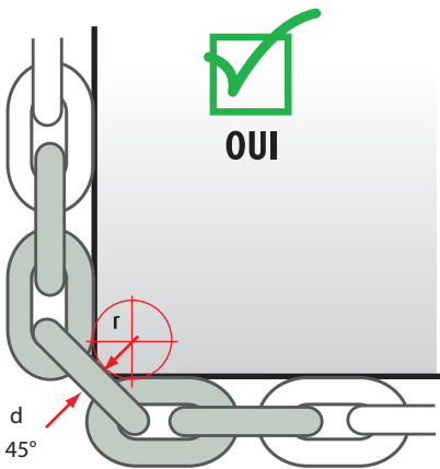
Figure 43 - Élingue chaîne sur arête vive
