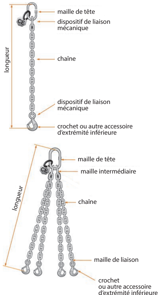
Figure 11 - Élingues chaînes
