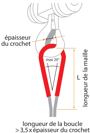
Figure 41 b - Dimension de la boucle d'extrémité
