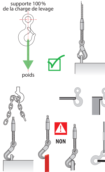
Figure 41 c - Utilisation du crochet
