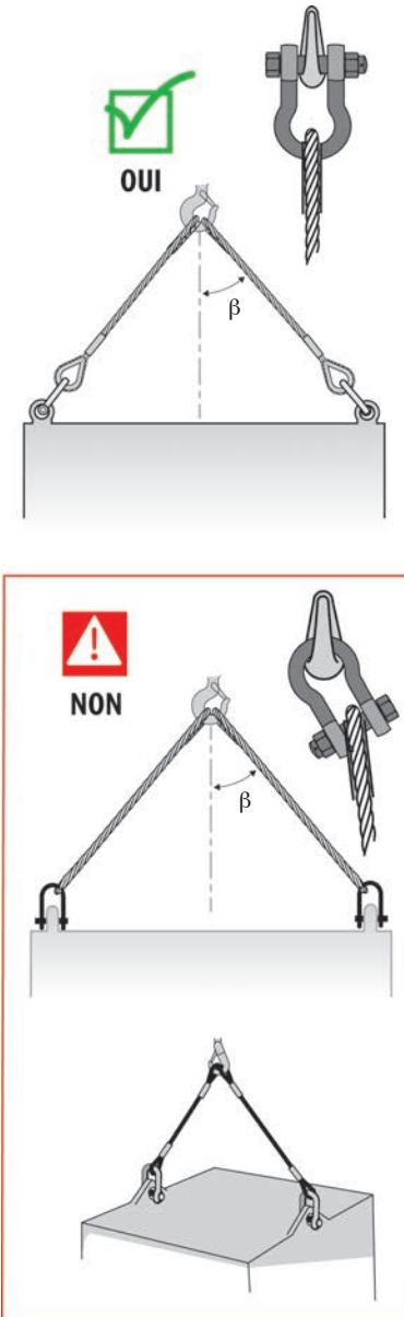
Figure 19 - Montage des manilles
