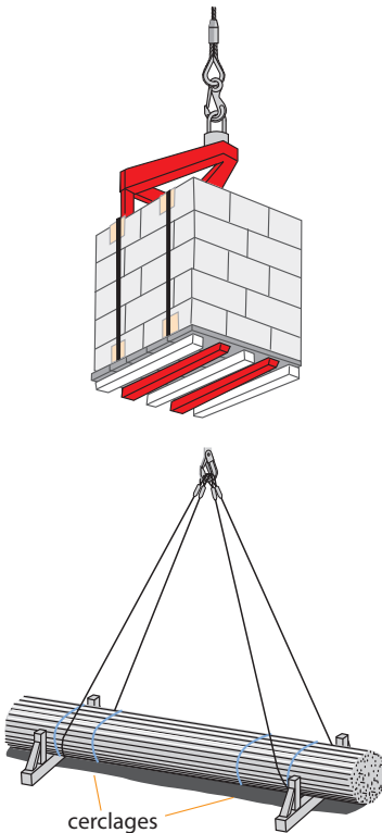
Figure 33 - Rendre les éléments de la charge solidaires
