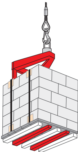
Figure 27 - Fourche à palette
