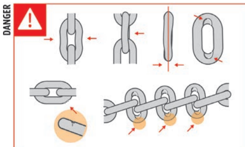
Figure 35 - Inspection des chaînes
