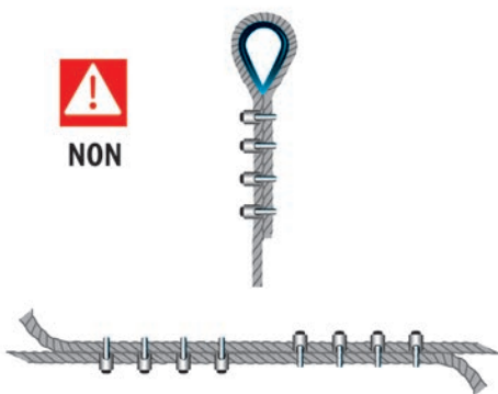
Figure 8 - Assemblages avec serre-câbles
