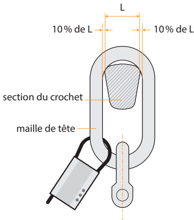
Figure 41 a - Dimension de la maille de tête
