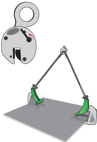
Figure 24 - Pince à tôle
